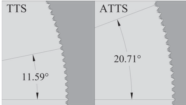
그림 5. TTS와 ATTS의 실접촉구간 비교 [Figure 5. Actual contact comparison TTS vs ATTS]
