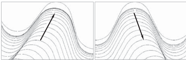
그림 2. 치형모의실험 [Figure 2. Tooth shape simulation]
