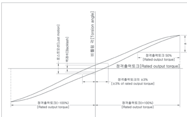
그림 7. 히스테리시스곡선 [Figure 7. Hysteresis curve]
