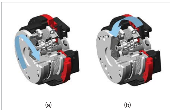
그림 8. Power 시리즈의 외부모멘트 하중 [Figure 8. Ext. moment load of Power series]
