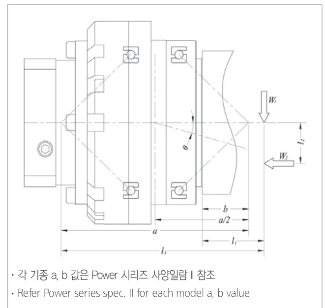
그림 9. 외부하중 작용선도 [Figure 9. External loading diagram]
